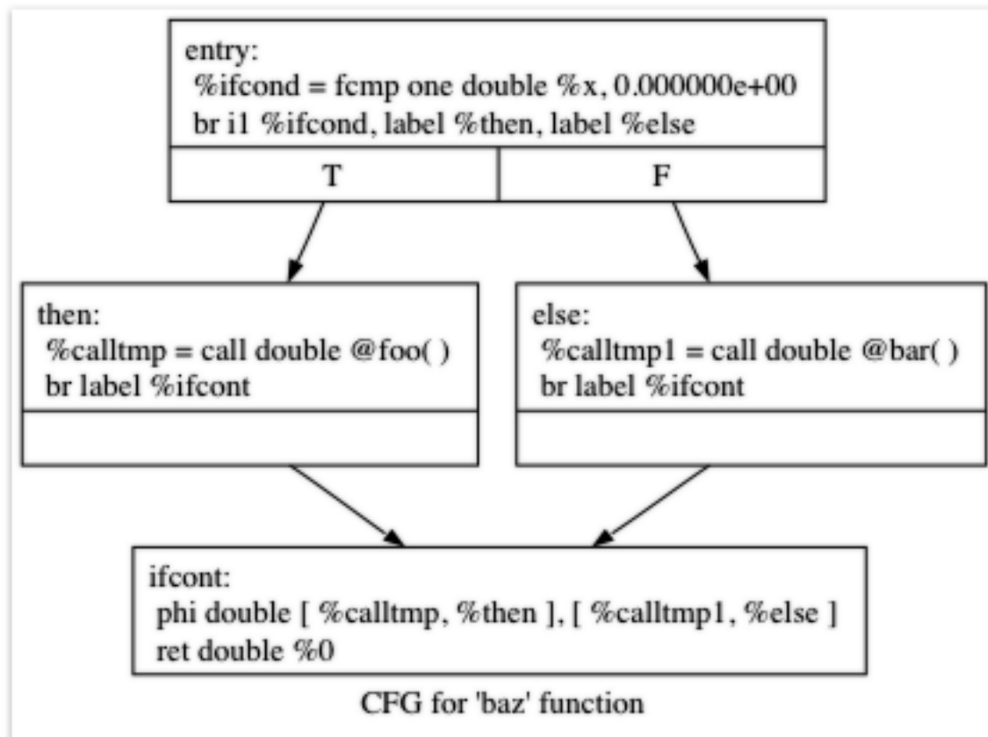
Fig. 2.1: Example CFG
